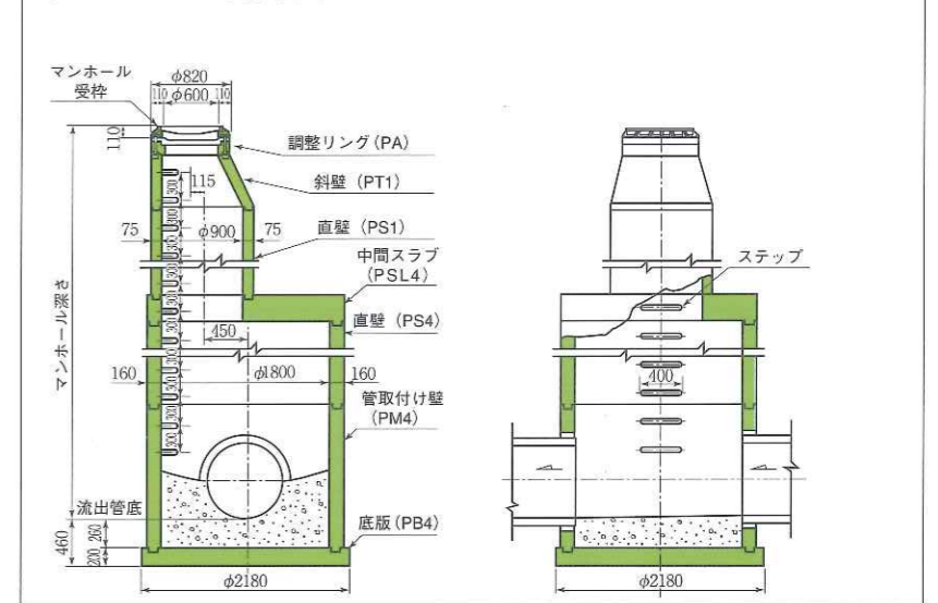
●プレホール4号標準図
