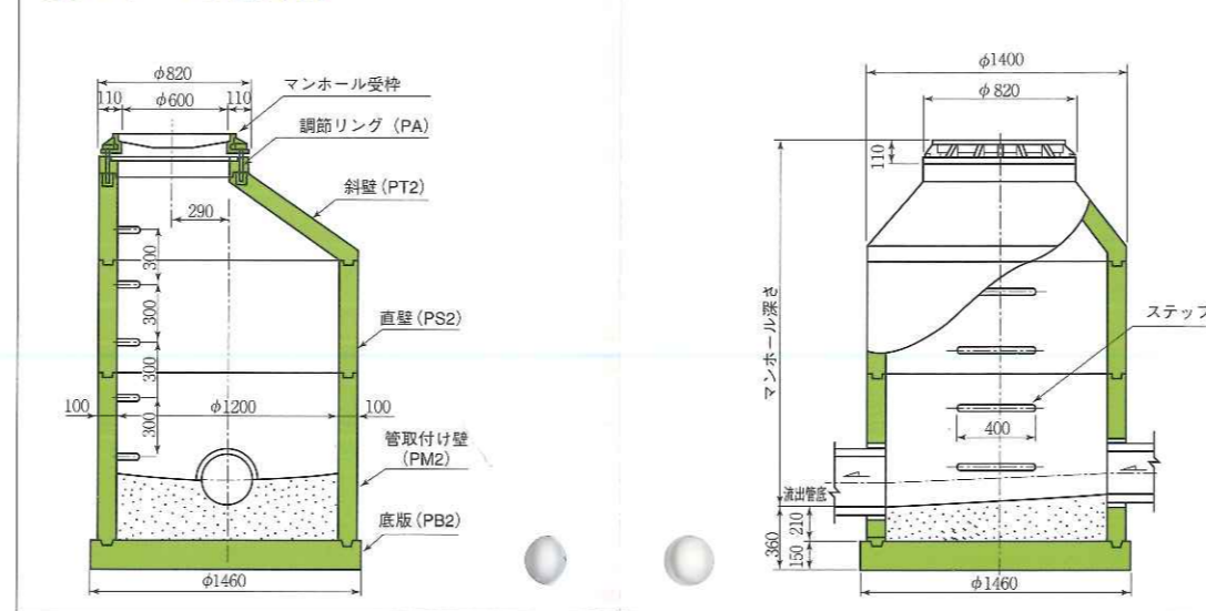
●プレホール2号標準図
