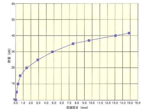
曲げ荷重と目地開きの関係
