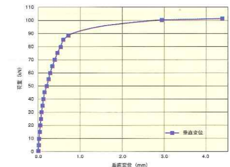
せん断荷重と垂直変位の関係
