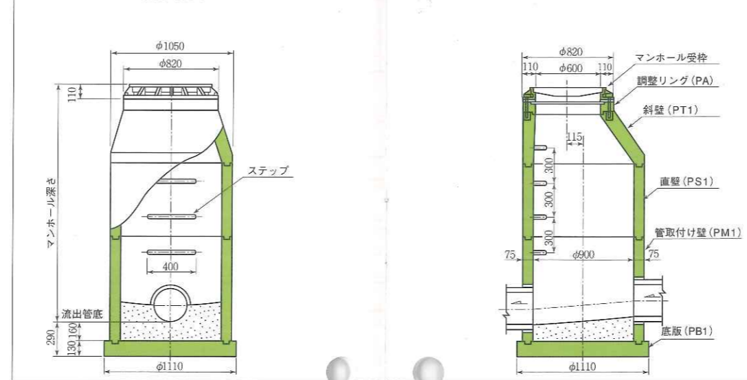
●プレホール1号標準図
