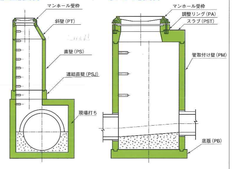
●連結直壁使用例
